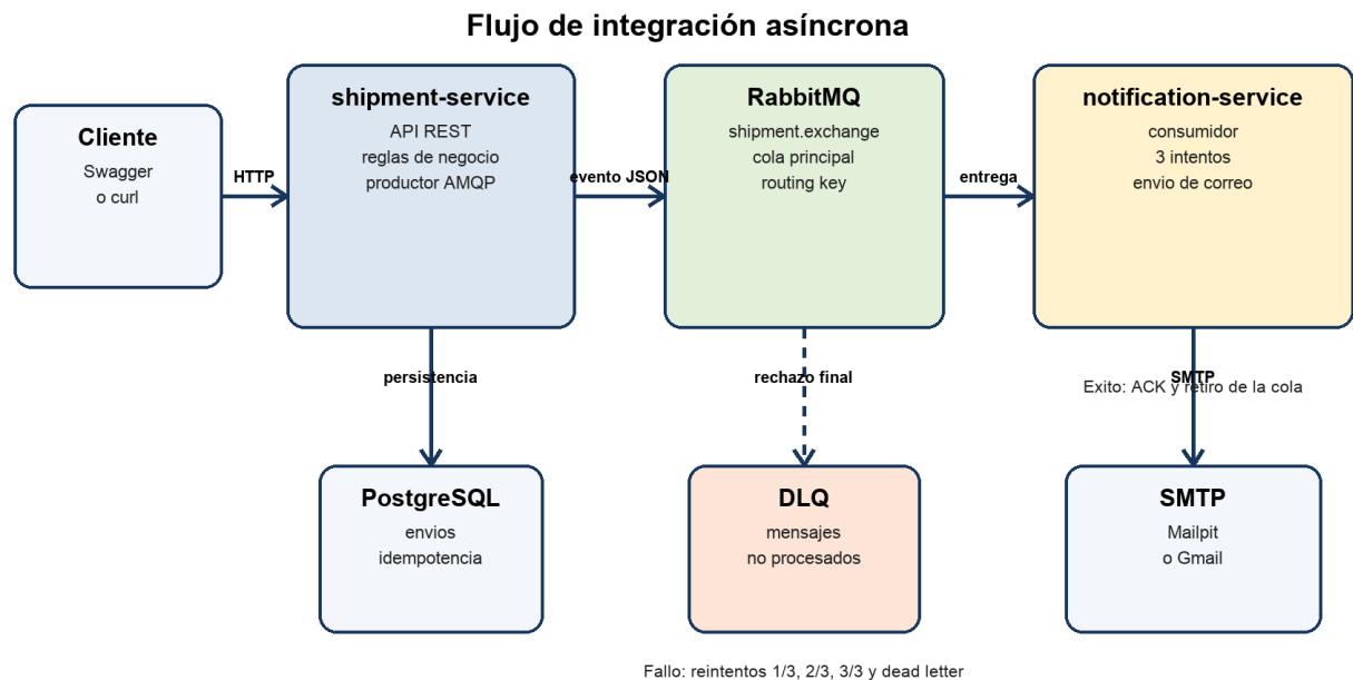
Figura 1 Arquitectura y flujo de mensajes del laboratorio
