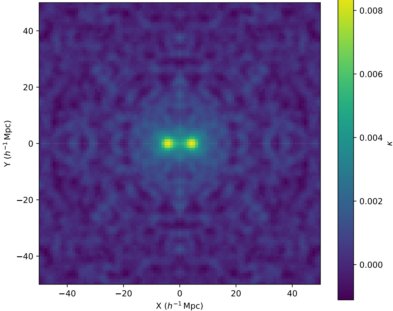
(2) Galaxy Pairs (10 Mpc/h)
