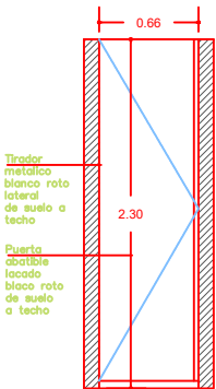
ALZADO EXTERIOR ARMARIO ROPA BLANCA
