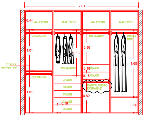
ALZADO INTERIOR ARMARIO HAB. PPAL
