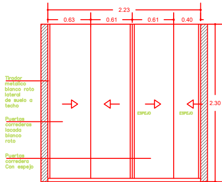
ALZADO ARMARIO PASILLO
