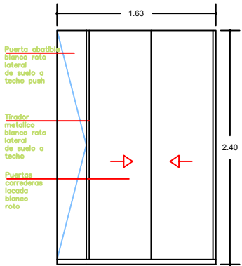
ALZADO EXTERIOR ARMARIO EMMA
