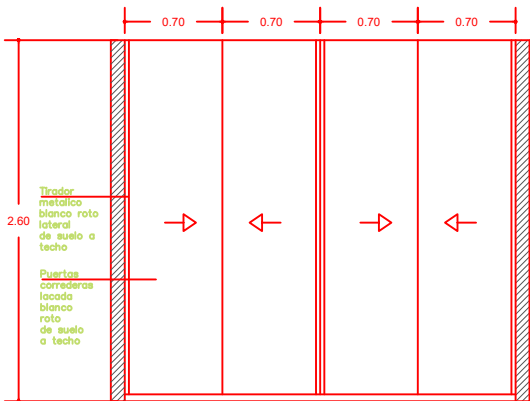
ALZADO EXTERIOR ARMARIO HAB. PPAL
