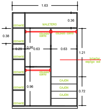
ALZADO INTERIOR ARMARIO EMMA
