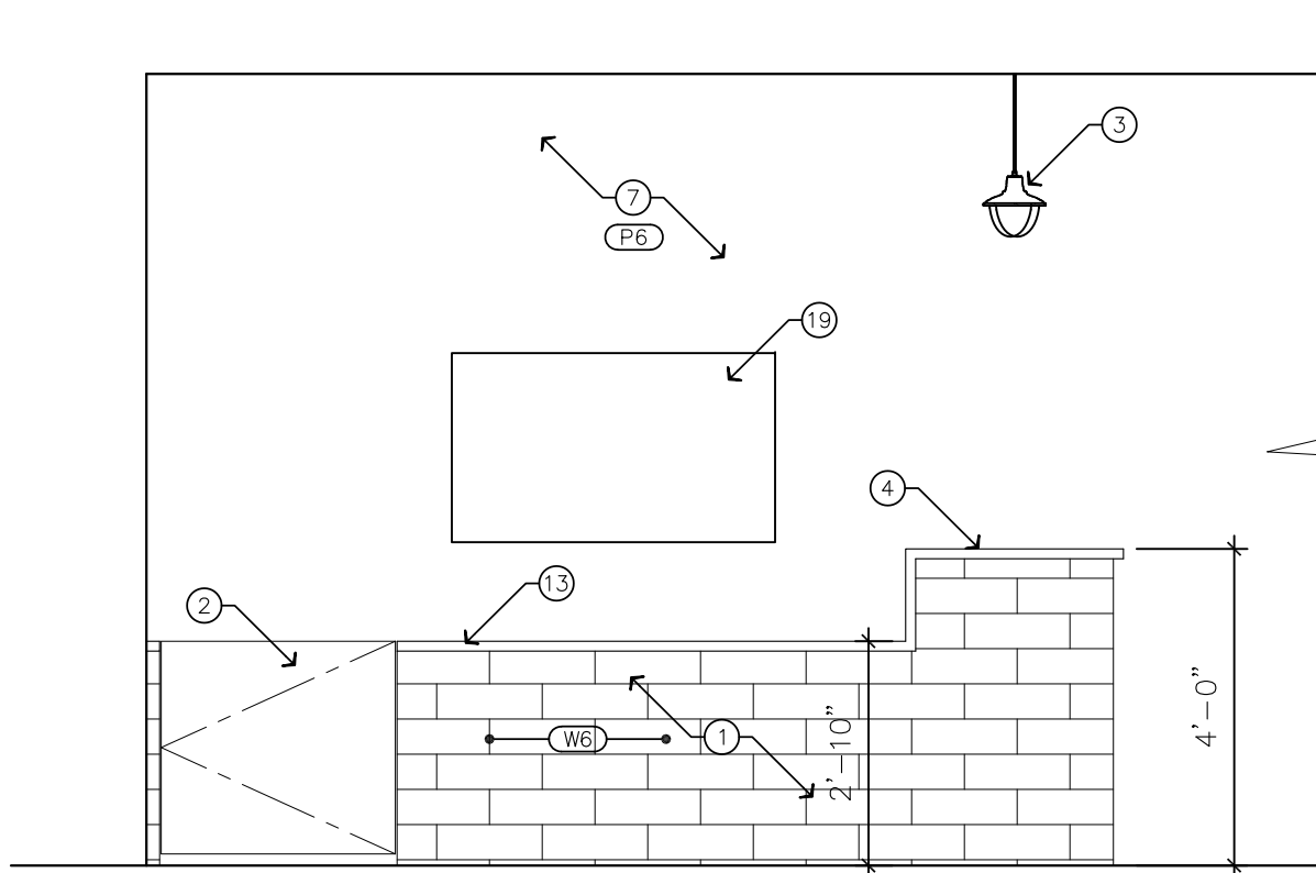
B ELEVATION
