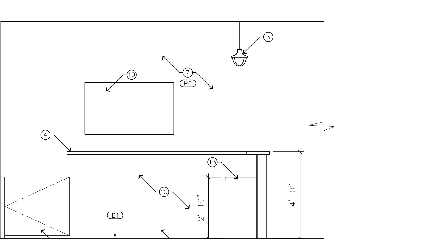
G ELEVATION
