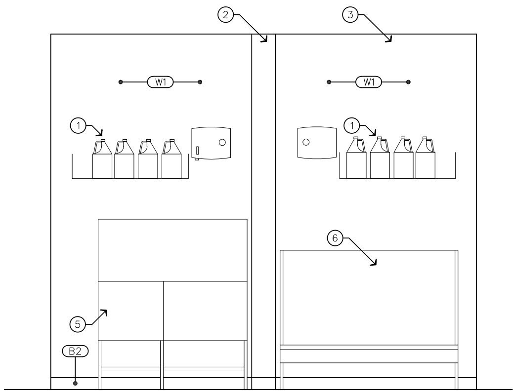
A ELEVATION
