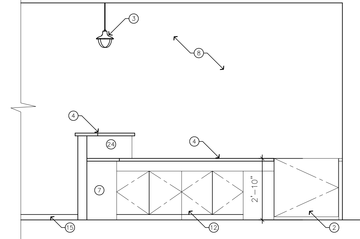
E ELEVATION
