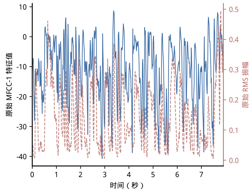
a 原始帧级序列
