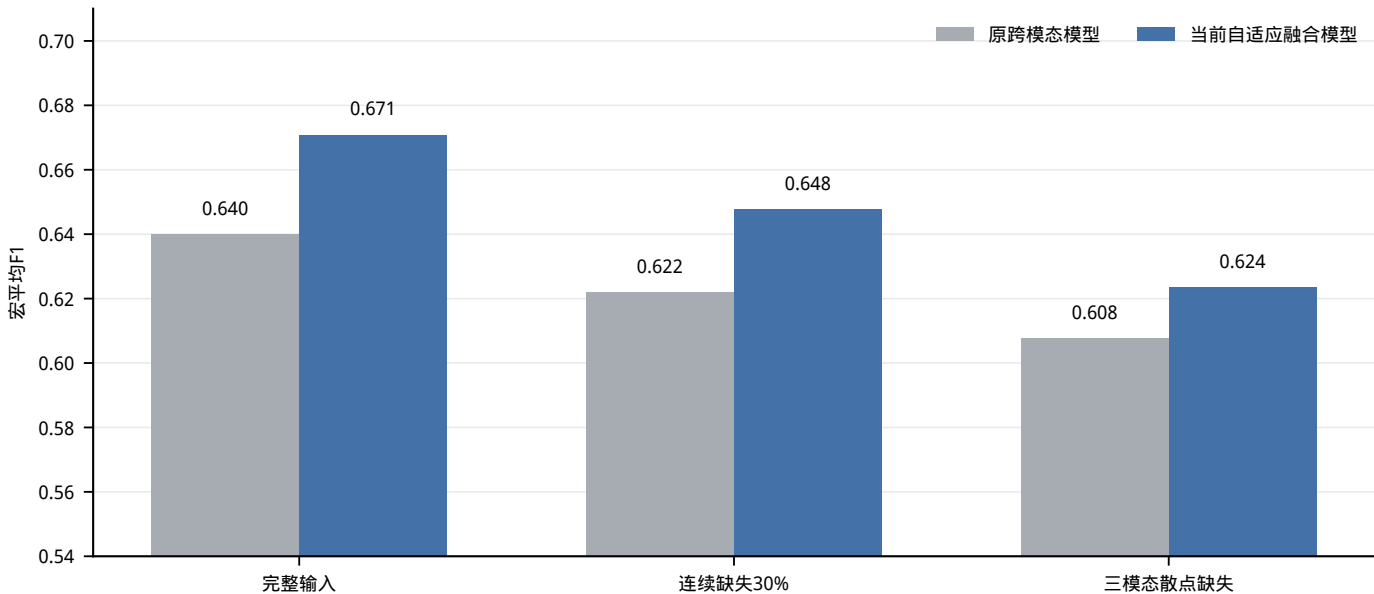
完整输入与模态缺失条件下的分类性能对比
