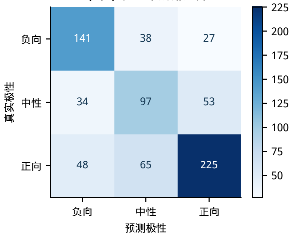
(甲) 验证集混淆矩阵
