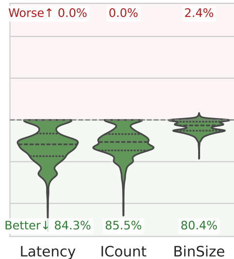
Model_Latency_3B vs -O0
