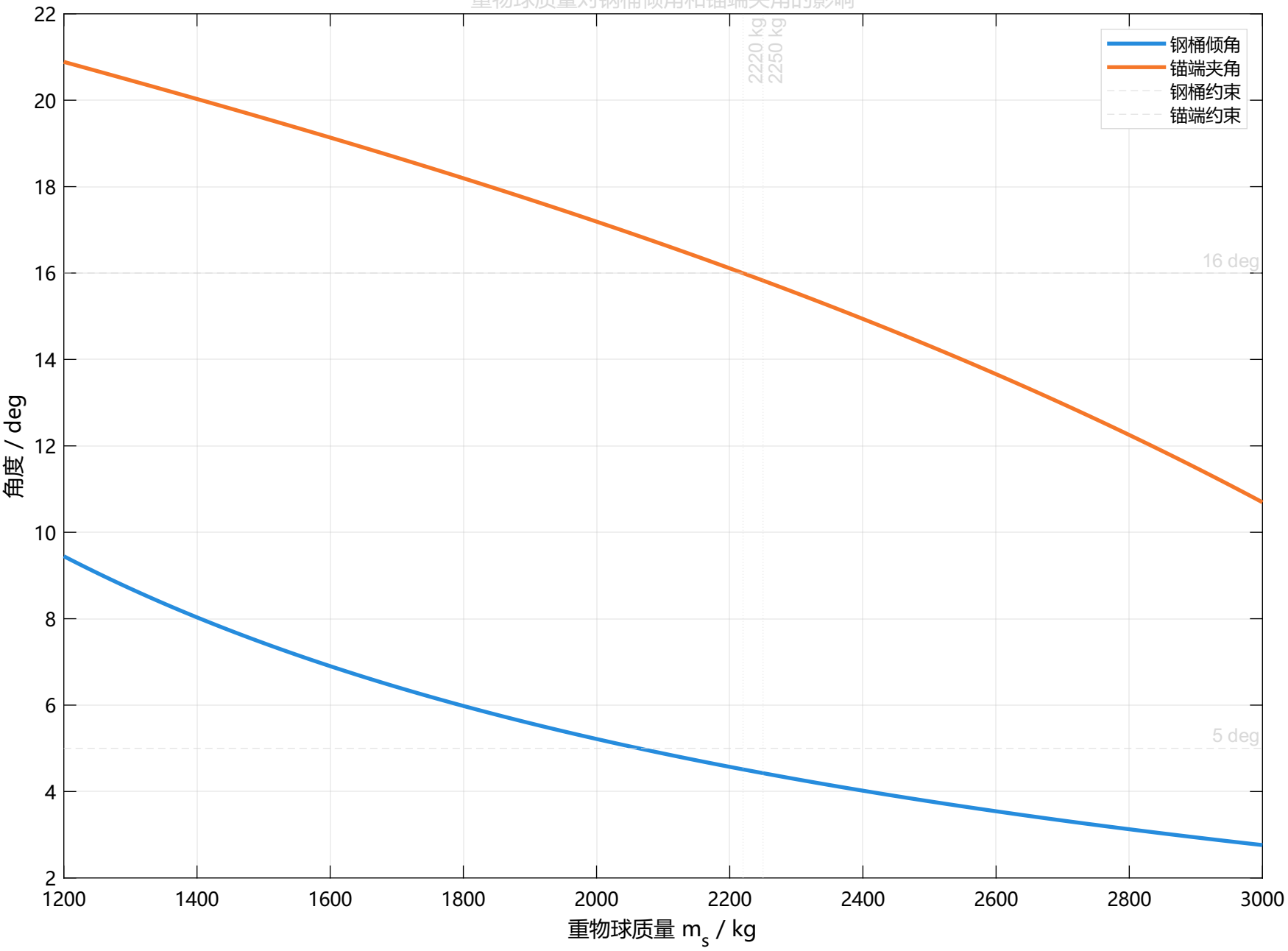
重物球质量对钢桶倾角和锚端夹角的影响
