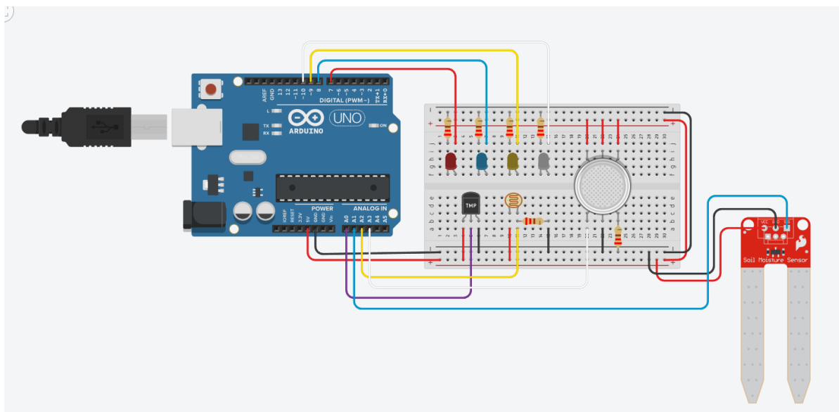
Figura 1 Escenario IoT simulado en Tinkercad – Arduino UNO con sensores y LEDs indicadores.
