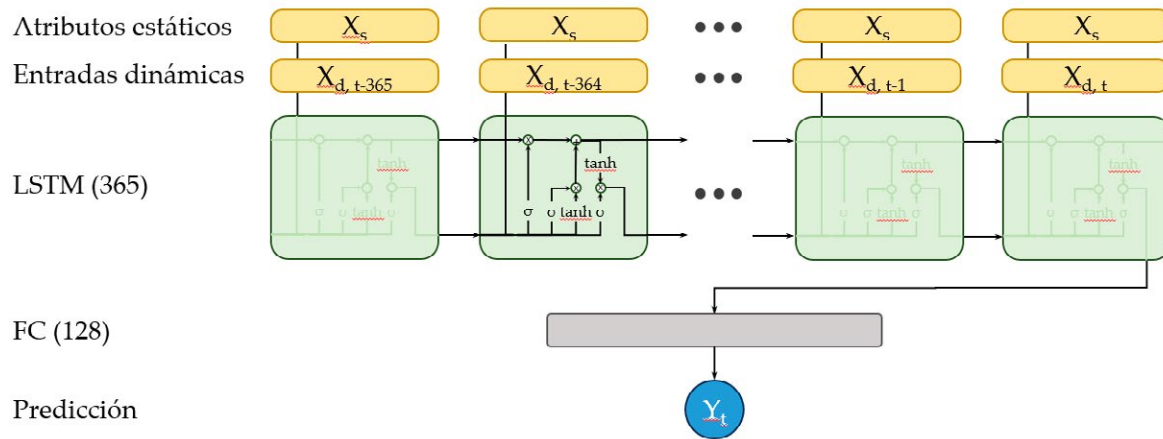
Figura 1 | Esquema de la red neuronal utilizada para predecir un dato diario de caudal ( Y_t ) a partir de los atributos estáticos de las cuencas ( X_s ) y las series temporales de los últimos 365 días ( X_d ). La red se compone de una red neuronal recurrente de tipo LSTM unida a una capa completamente conectada (FC).
