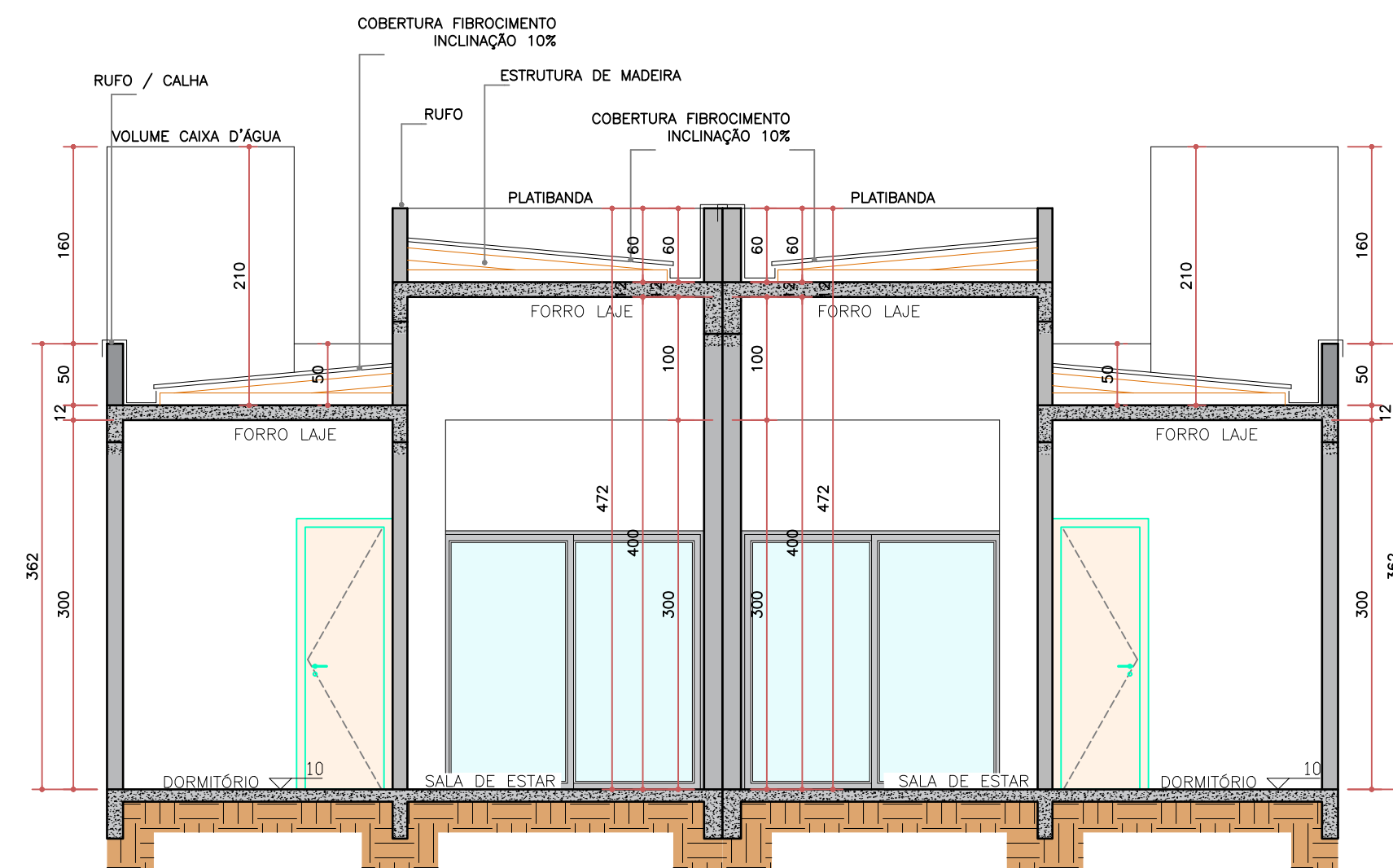
CORTE A1 ESCALA: 1/50
