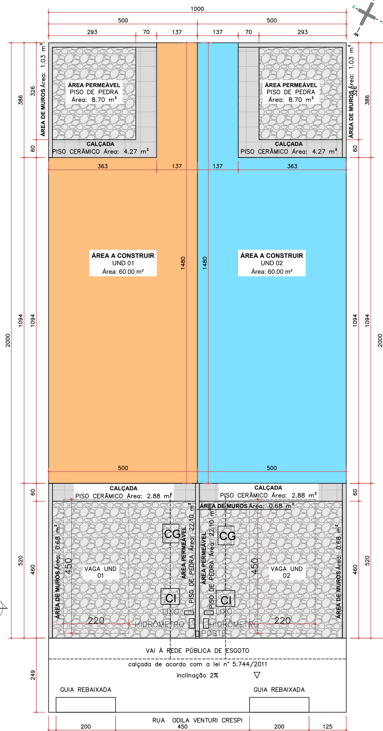
SITUAÇÃO ESCALA: 1/75
