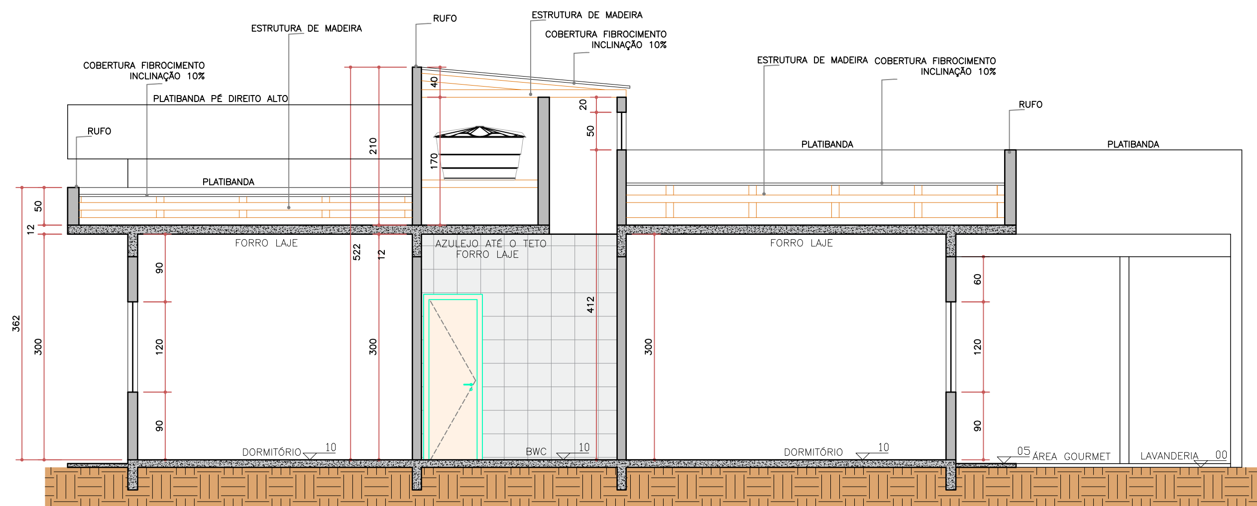
CORTE B1 ESCALA: 1/50
