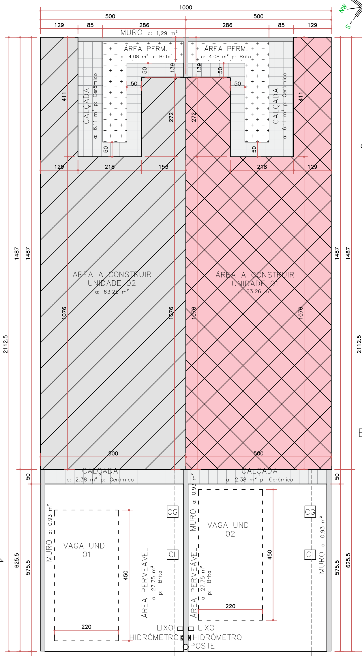
calçada de acordo com a lei nº 5.744/2011 piso antiderrapante 1:2% 25 200 450 200 125 GUIA REBAIXADA R. JOSÉ NUNES SITUAÇÃO ESCALA: 1/75
