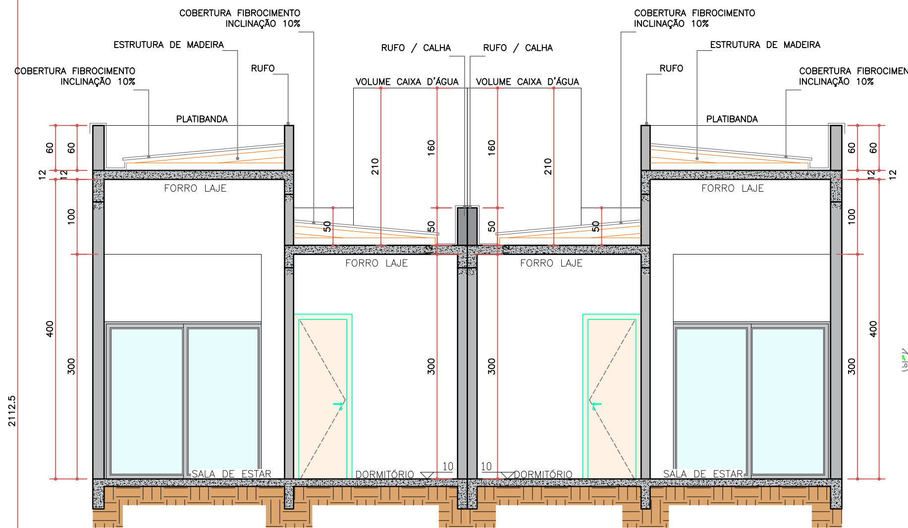
CORTE A1 ESCALA: 1/50
