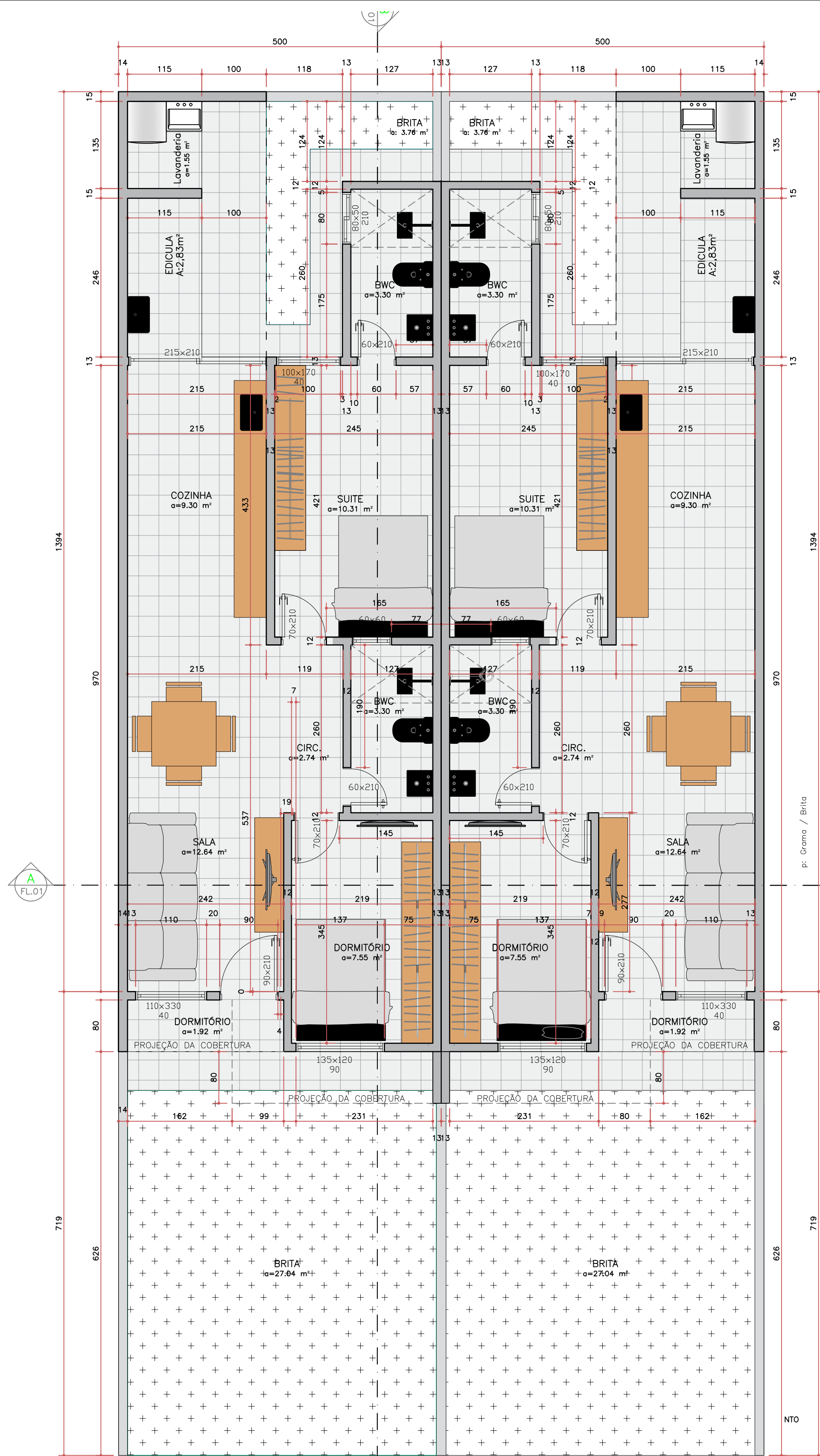
PLANTA BAIXA ÁREA: 63,26m 2
