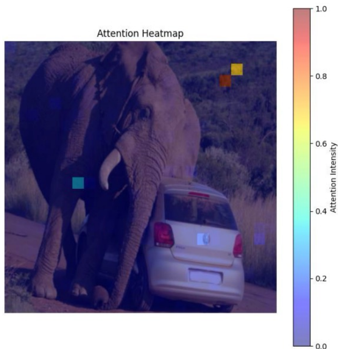
CLIP-ViT
