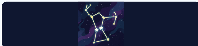
Orion
