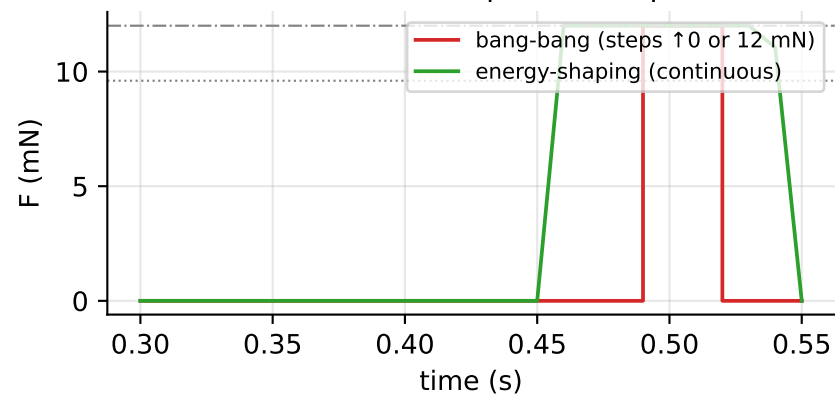
(d) zoom on one hop — thrust profile
