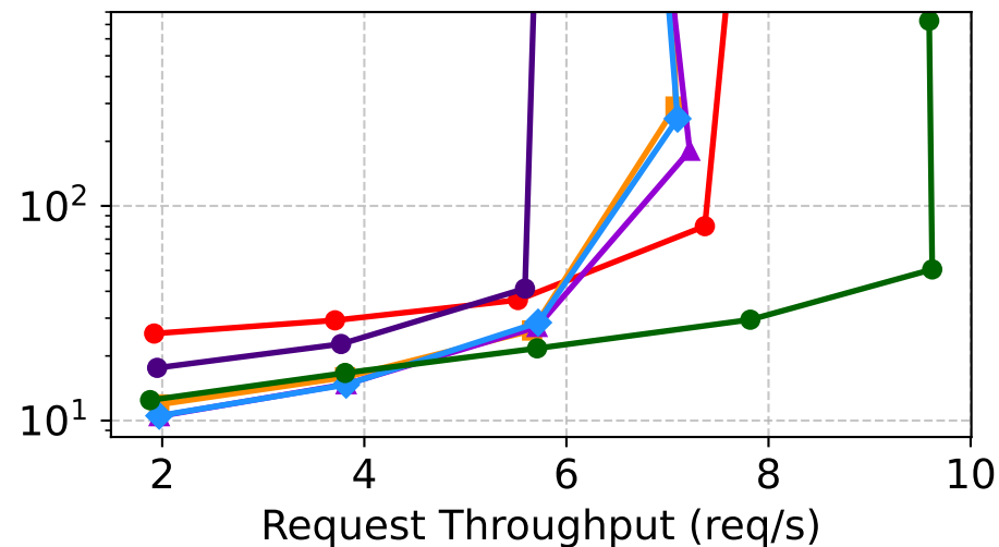
(e) OPT-30B / OPT-350M
