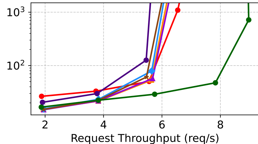
(c) OPT-13B / OPT-125M
