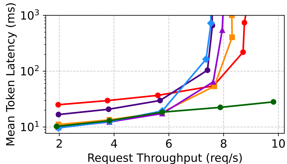
(a) OPT-6.7B / OPT-125M
