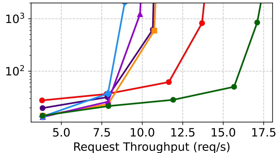
(b) Llama-13B / Vicuna-68M
