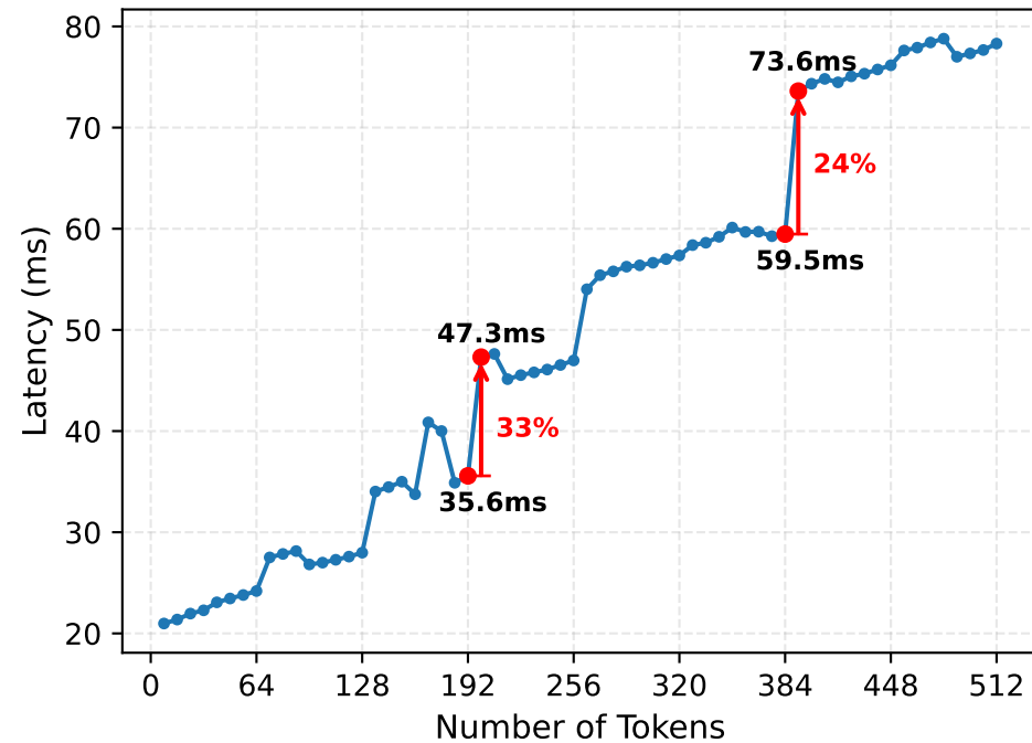
Model: OPT-6.7B / GPU: A6000
