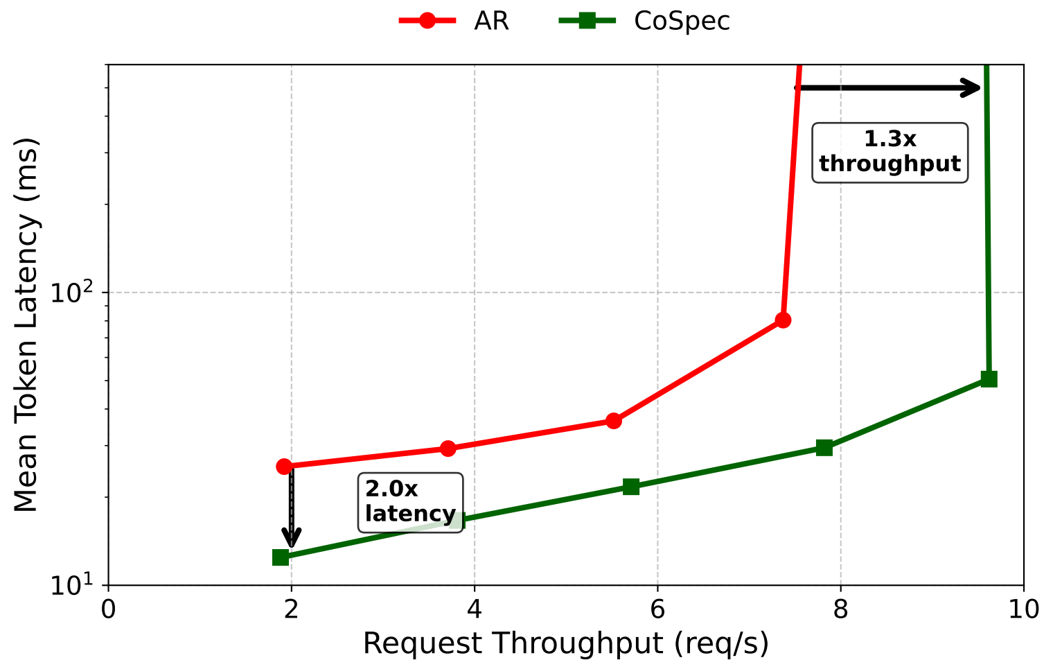
(e) OPT-30B/OPT-350M (H200)
