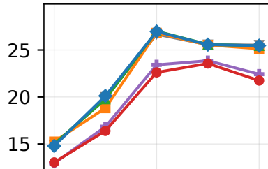
Qwen3-30B-A3B
