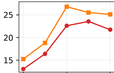
Qwen3-30B-A3B
