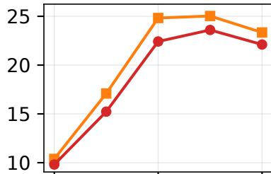
Gemma-4-26B-A4B
