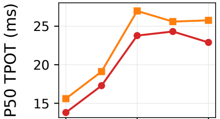
Qwen3-30B-A3B
