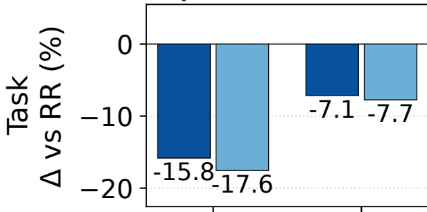
Qwen3-30B-A3B
