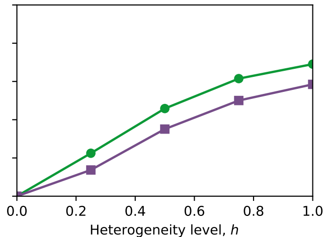
(d) JR timescale: q
