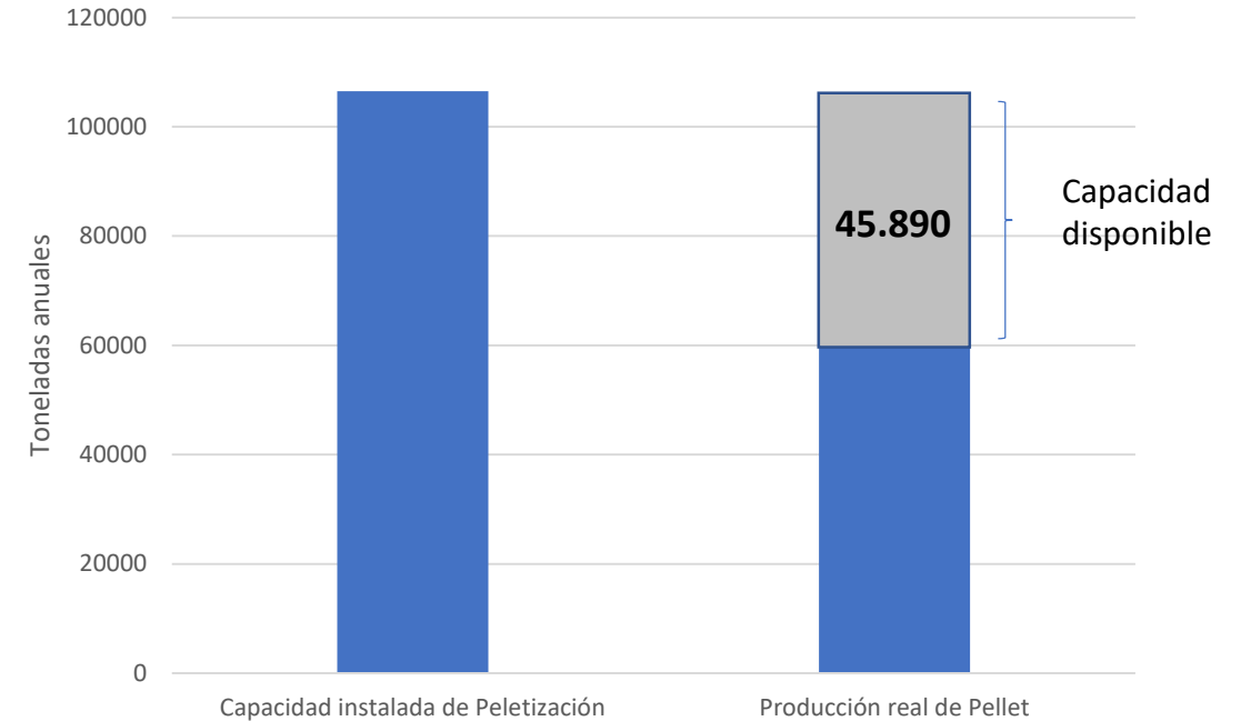
Capacidad instalada de peletización v/s producción pellets
