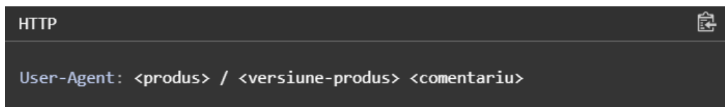
Figura 2.1: Sintaxa user-agent-ului
