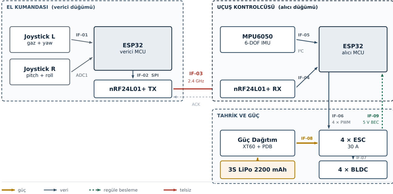
Şekil 4.2 — İç blok diyagramı. Kalın oklar güç, ince oklar veri akışını gösterir. Port etiketleri fiziksel arayüzü belirtir.
