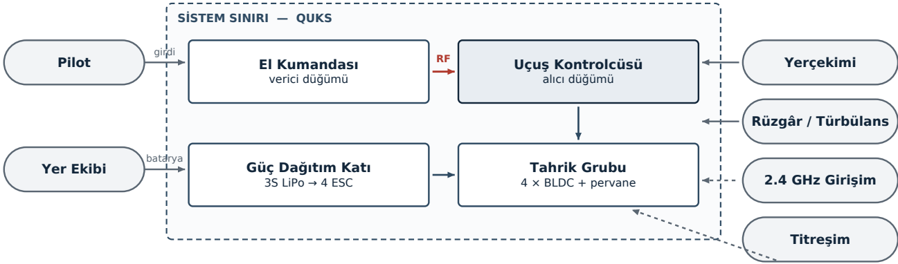
Şekil 2.1 — Sistem bağlam diyagramı. Kesikli çerçeve sistem sınırını, dış kutular sistemle etkileşen aktör ve etkenleri gösterir.
