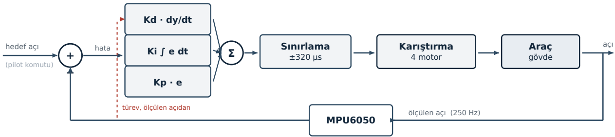
Şekil 8.1 — Tek eksen kapalı çevrim blok şeması. Türev terimi hata yerine ölçülen değerden alınır (derivative-on-measurement).
