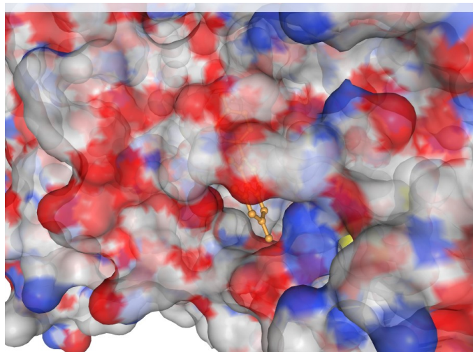
Gambar 4. Pose docking terbaik Genistein pada Cavity 1 PPARG (1PRG) — permukaan elektrostatik hasil CB-Dock2, menunjukkan ligan (oranye) menempati ligand-binding pocket.
