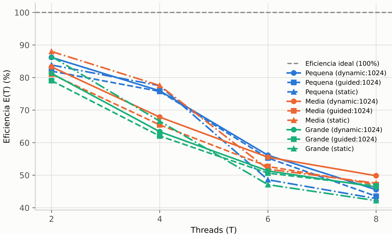
Eficiencia em funcao do numero de threads
