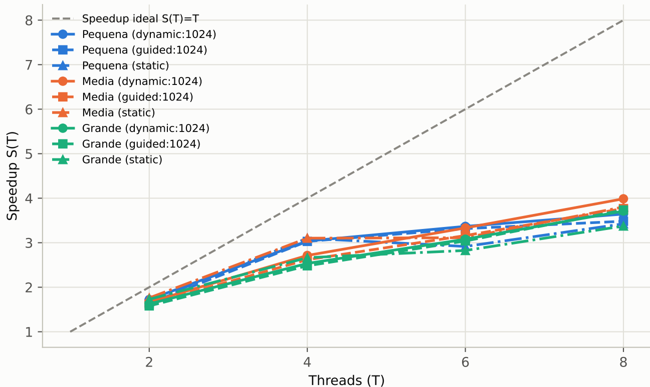
Speedup em funcao do numero de threads
