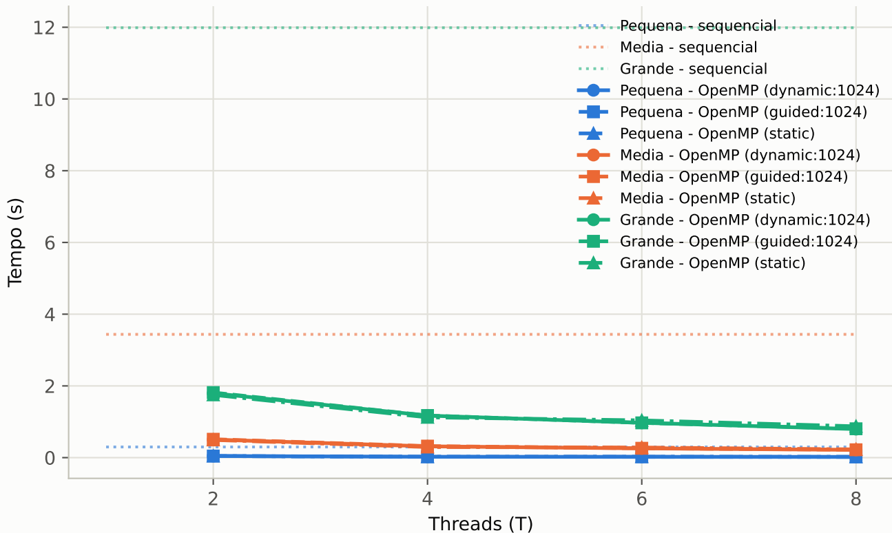
Tempo de execucao em funcao do numero de threads
