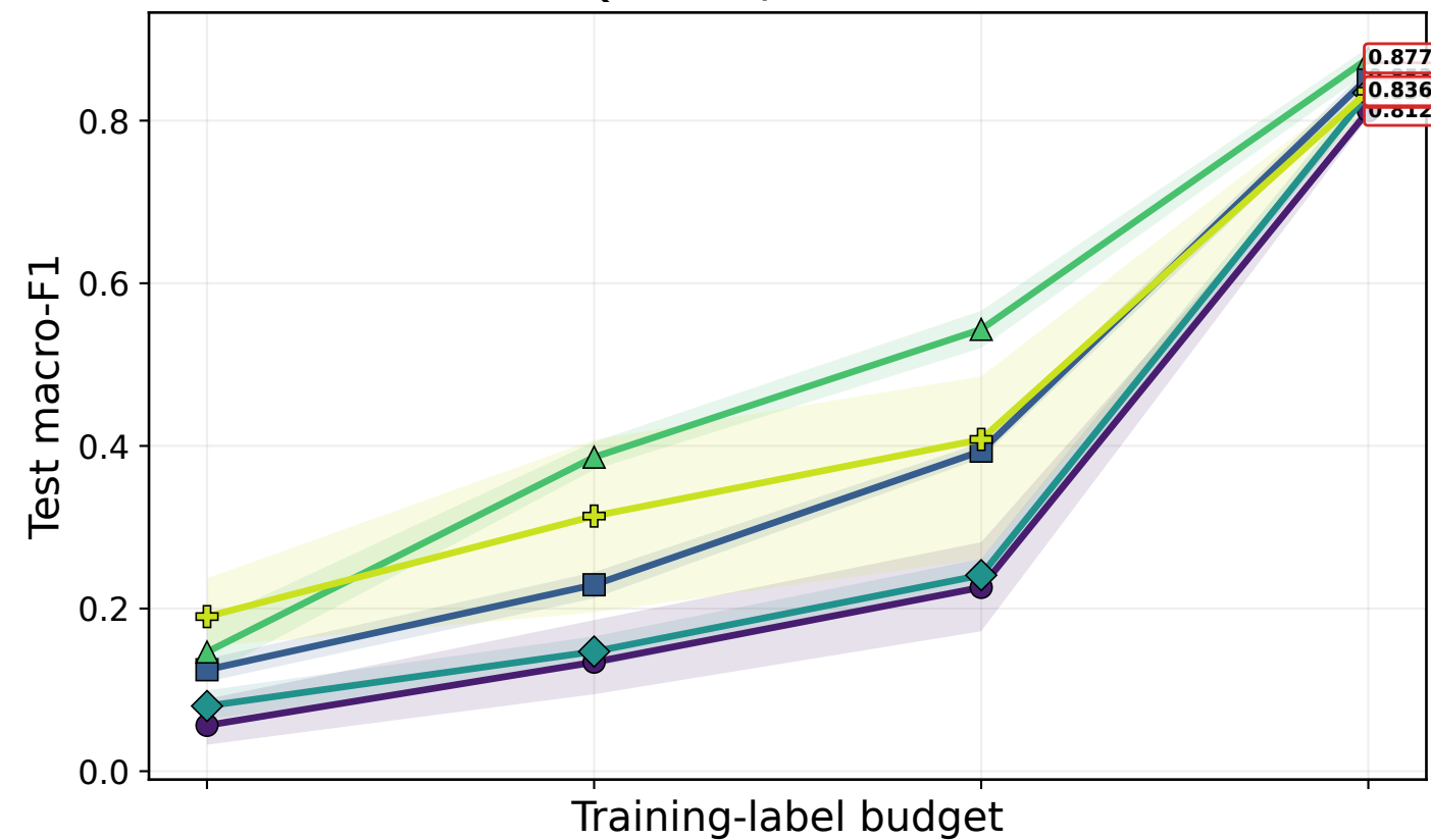
AQUA20 / DINOv2-S
