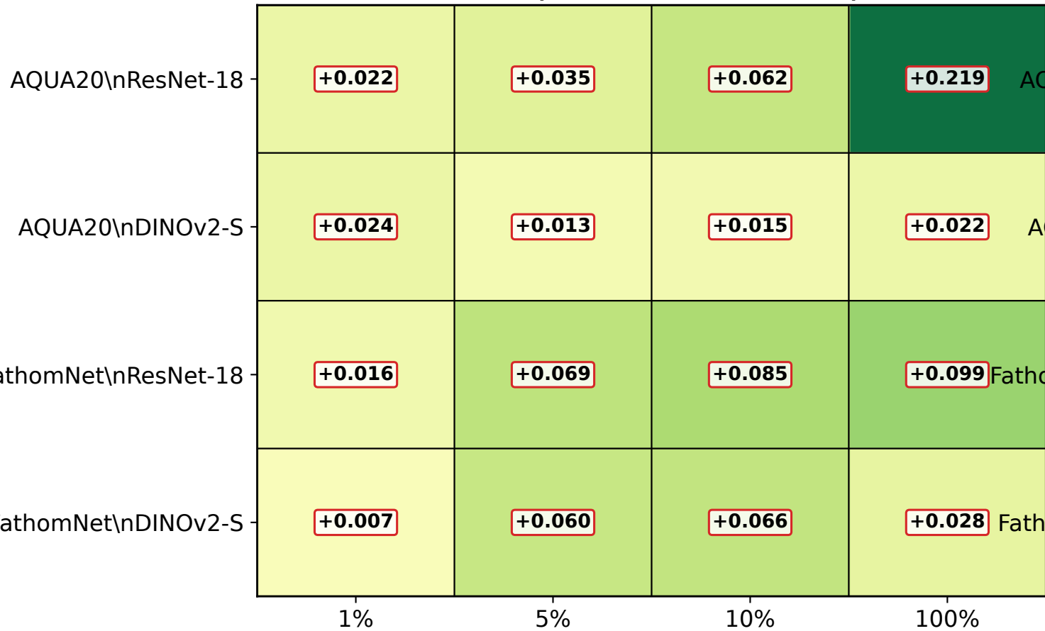
MarineAdapter minus Linear probe
