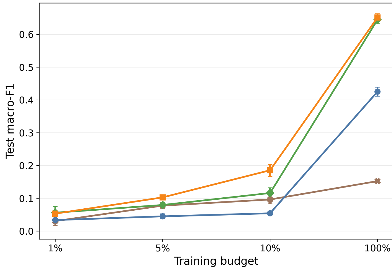
AQUA20
