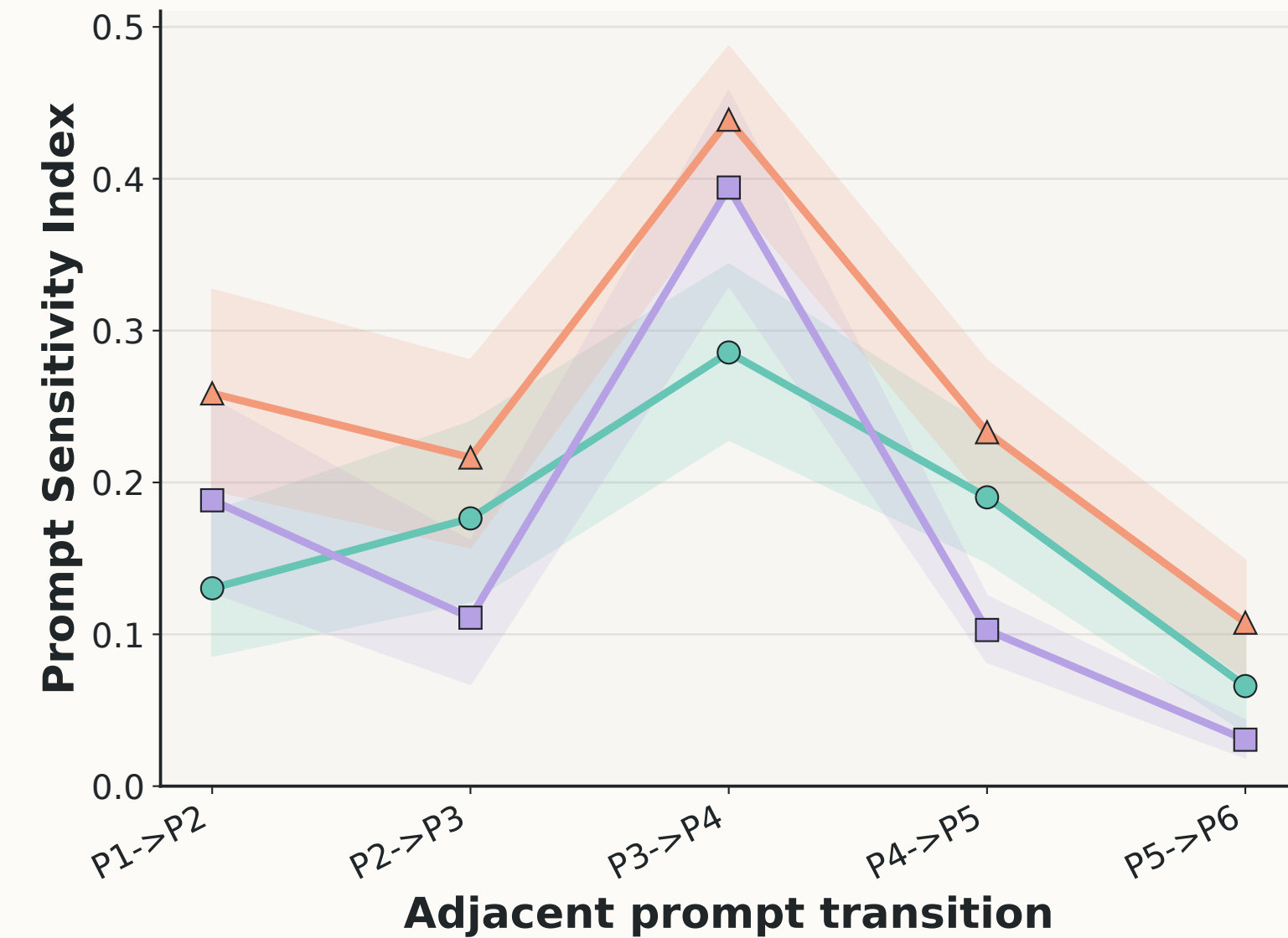
SciERC
