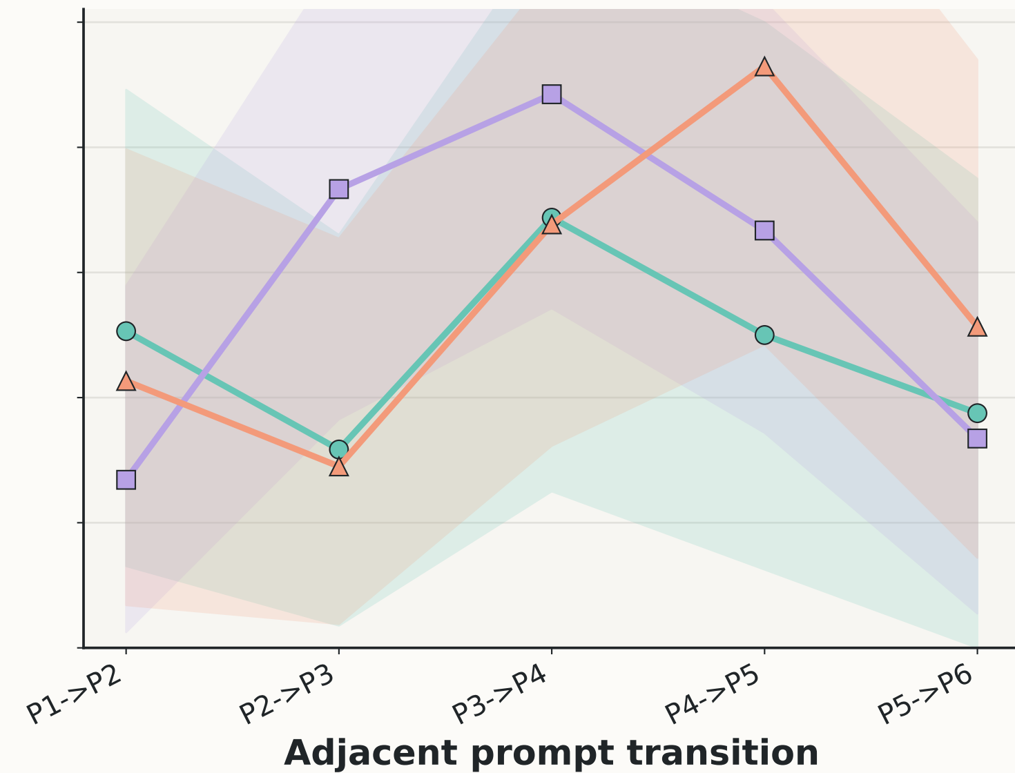
SciER
