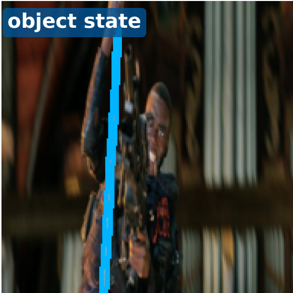
Input t-0
