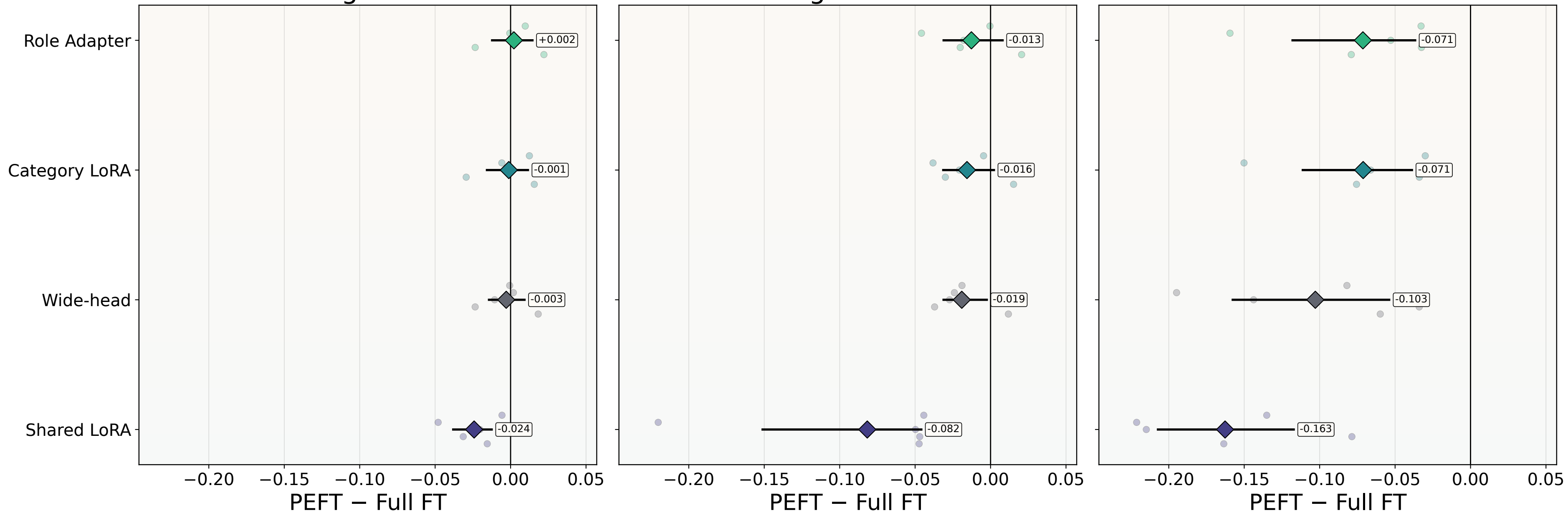
InLegalBERT
