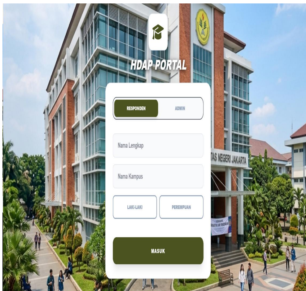
Gambar 2 Login Page
