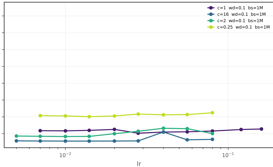
60M — muon
