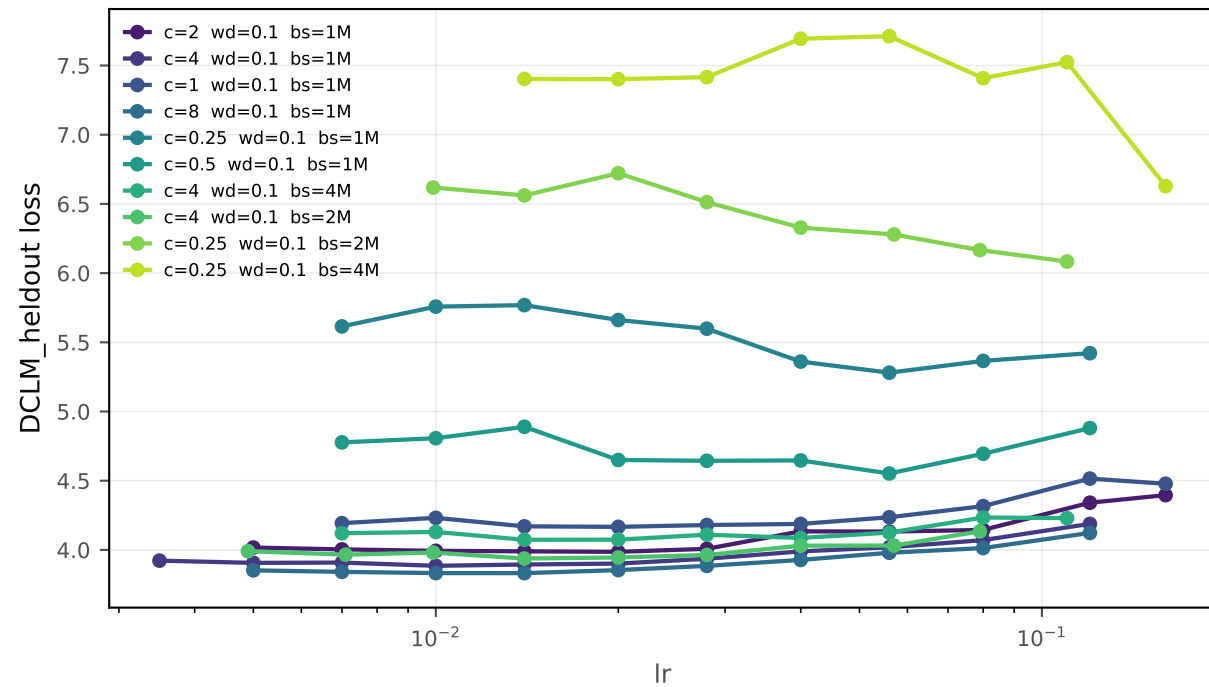
60M — adamw
