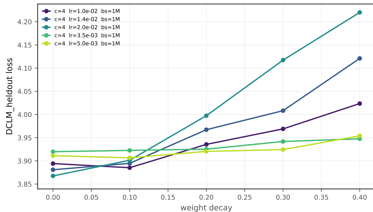
60M — adamw
