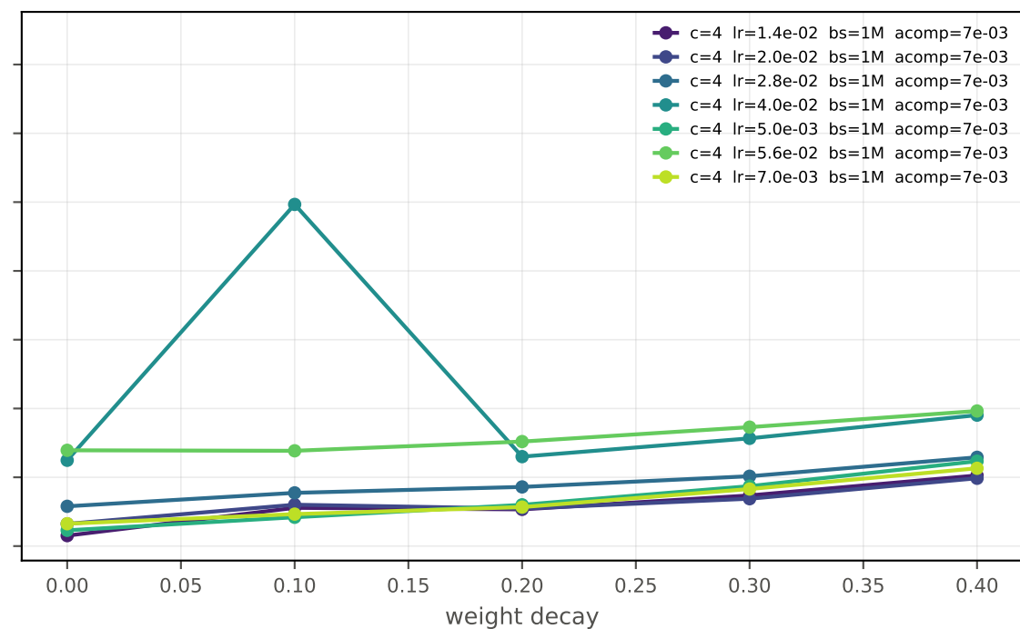
60M — muon
