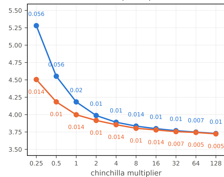
60M (0.06B)
