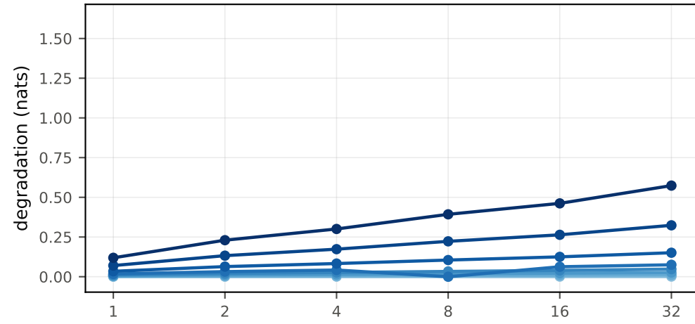
60M (0.06B) — adamw
