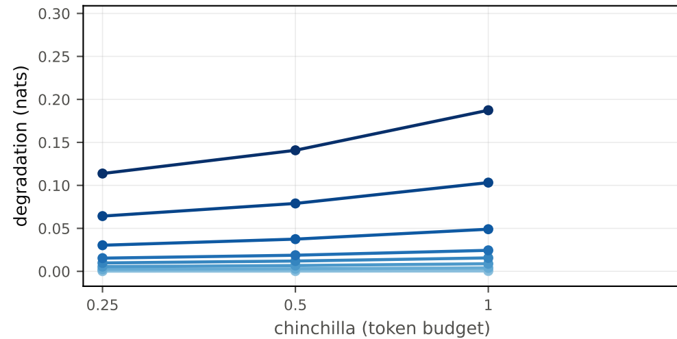
600M (0.6B) — adamw
