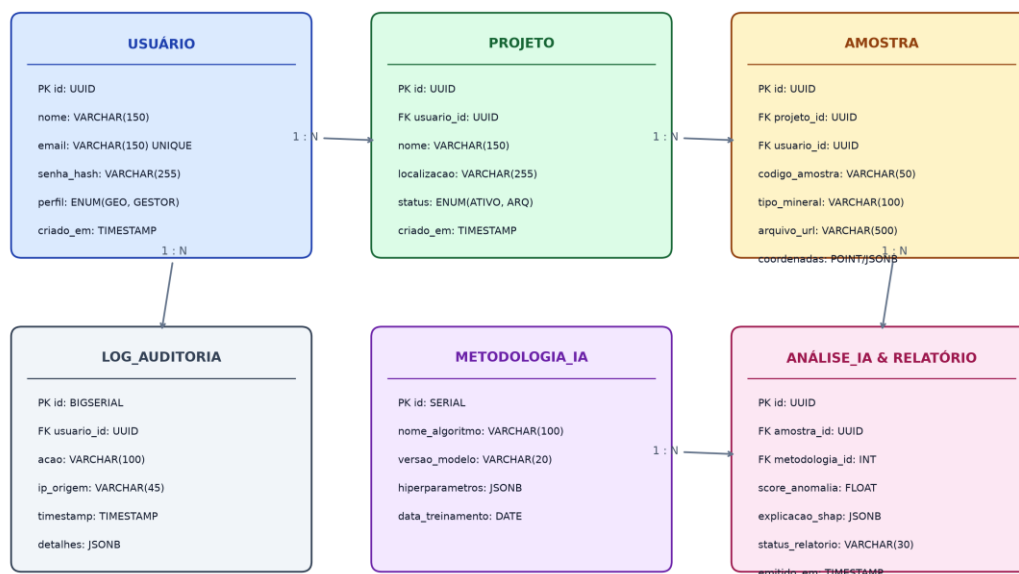
Figura 2 – Modelo Lógico de Dados (DER normalizado em 3FN) do Sistema OrenAI.
