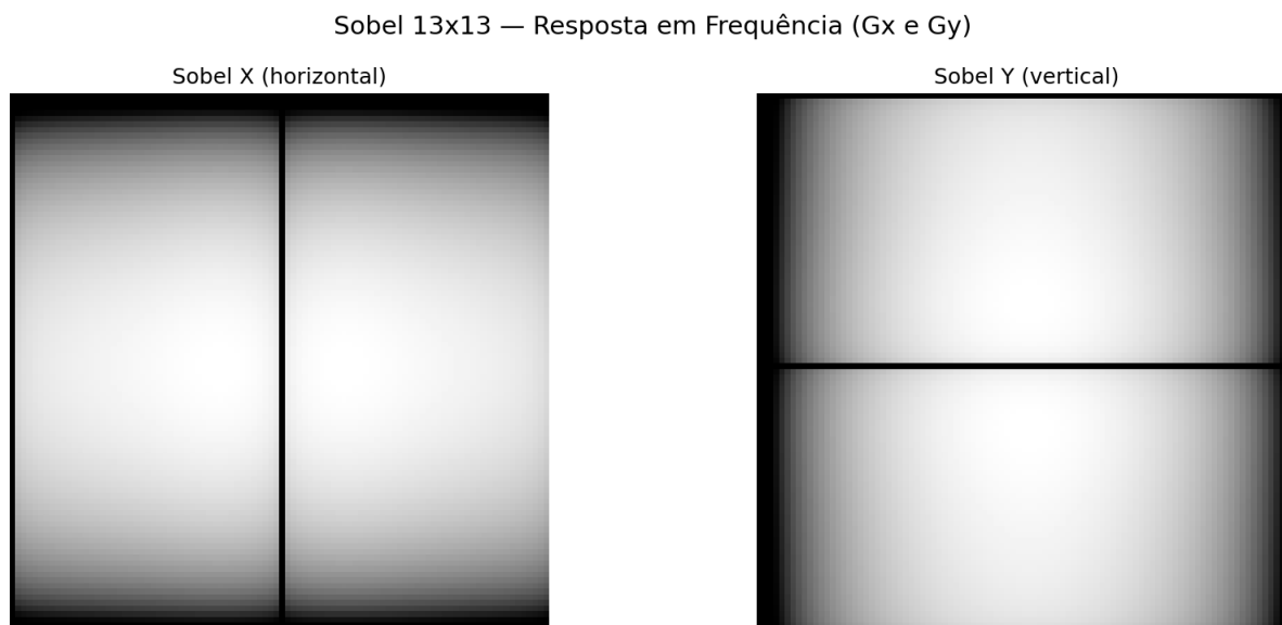
Figura 22: Sobel: resposta dos kernels
