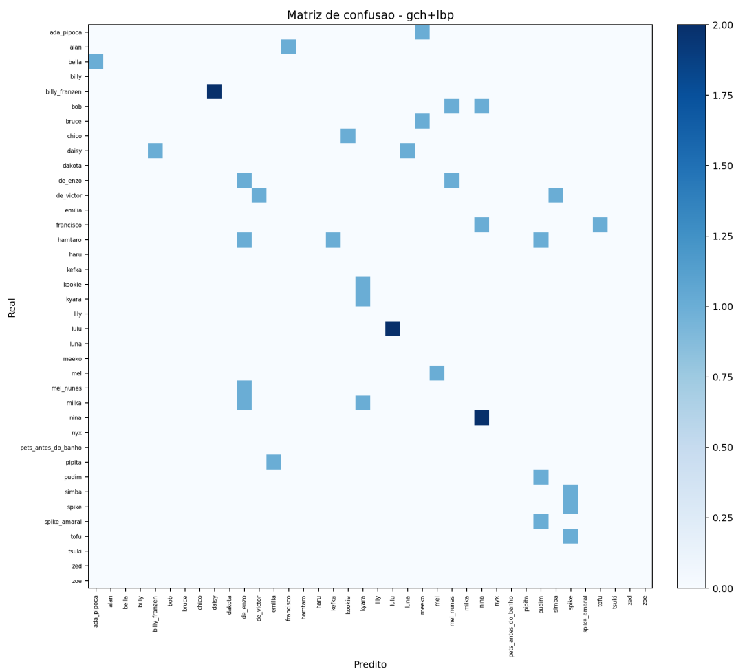
Figura 16: Matriz de confusão completa para GCH+LBP.
