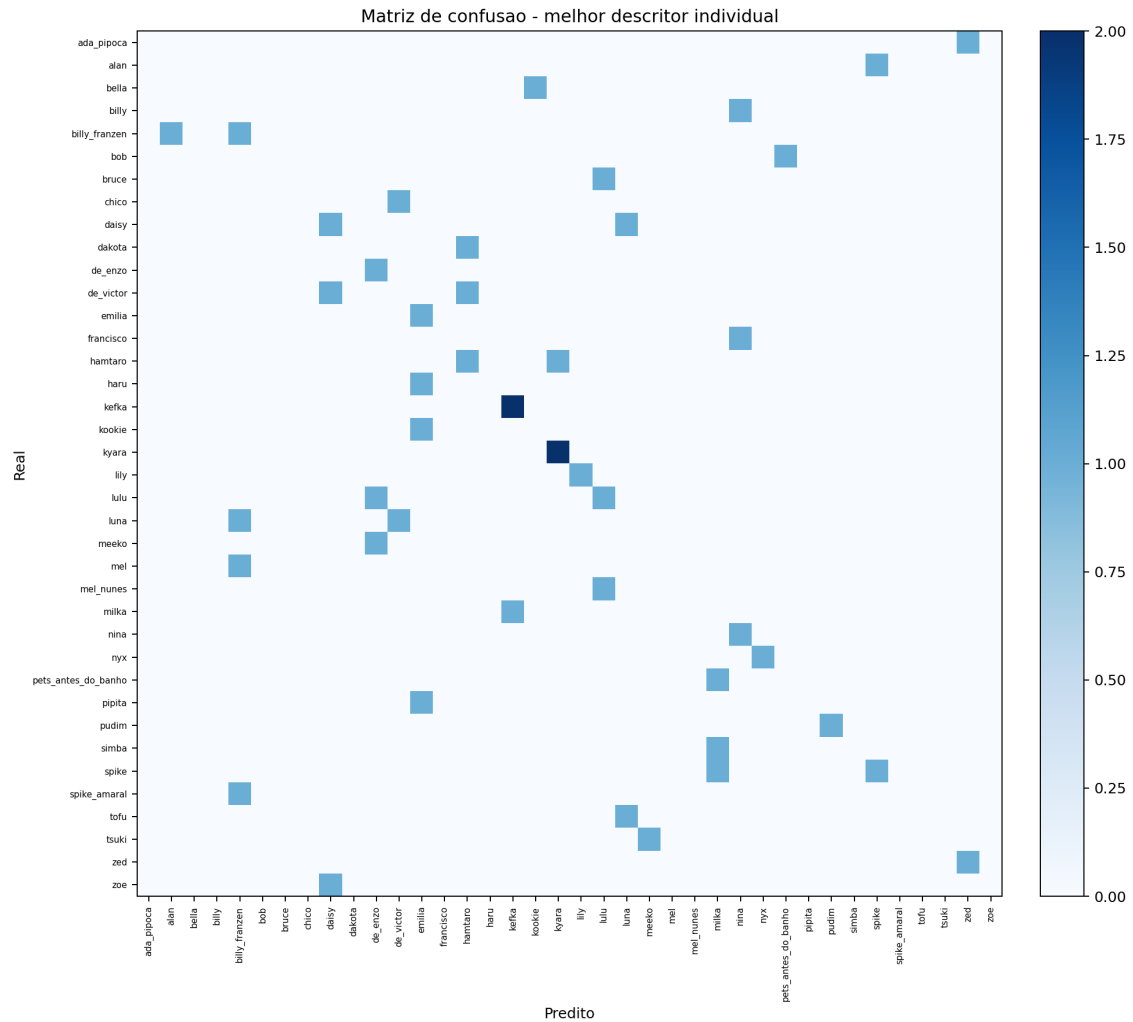
Figura 2: Matriz de confusão para o melhor descritor individual.
