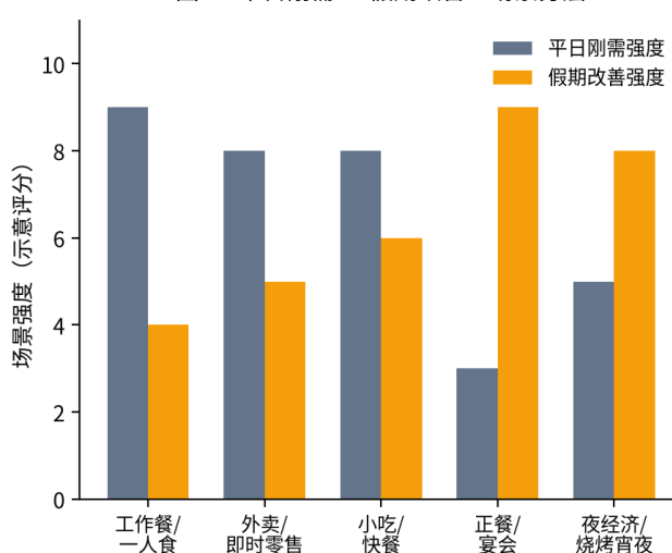
图4b 平日刚需 vs 假期改善：场景分层
