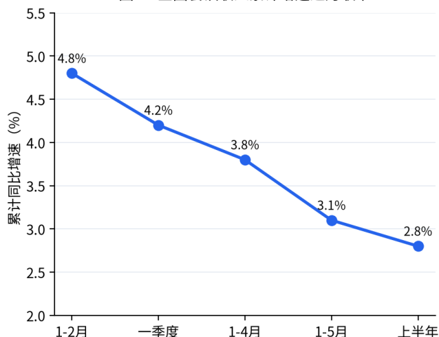
图4a 全国餐饮收入累计增速逐月收窄
