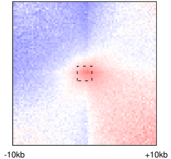
ED (n=179333)
