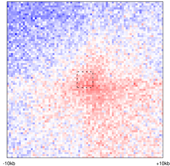
WD (n=5116)
