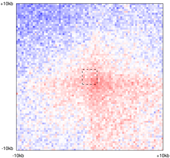
Embryo (n=5116)
