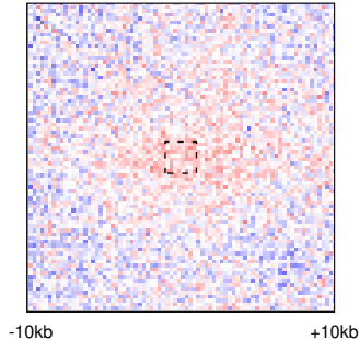
ED (n=2839)
