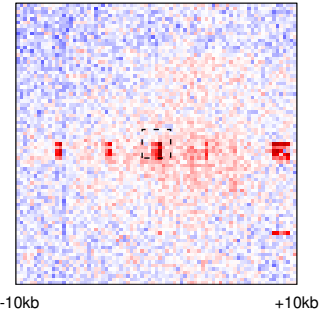
Embryo (n=2839)
