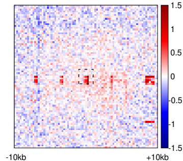
WD (n=2839)
